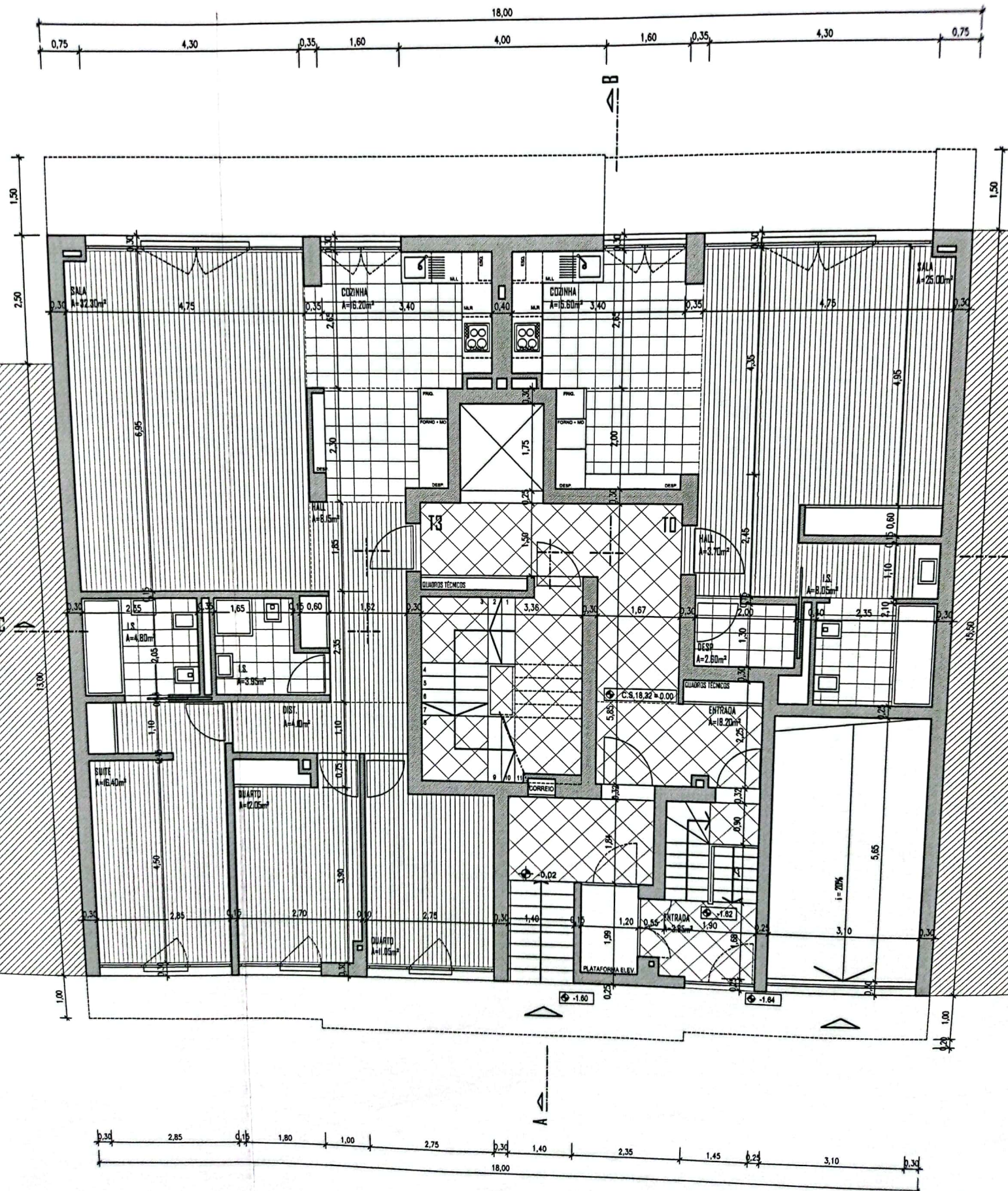
PLANTA PISO 0
