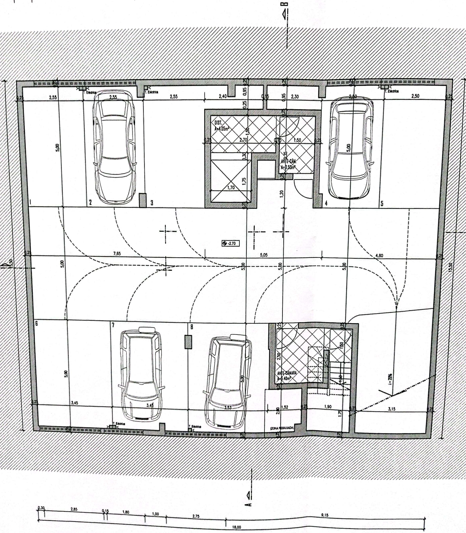
PLANTA PISO -1
