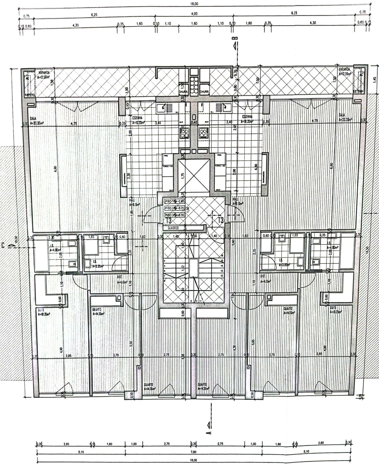
PLANTA PISOS 1, 2 e 3
