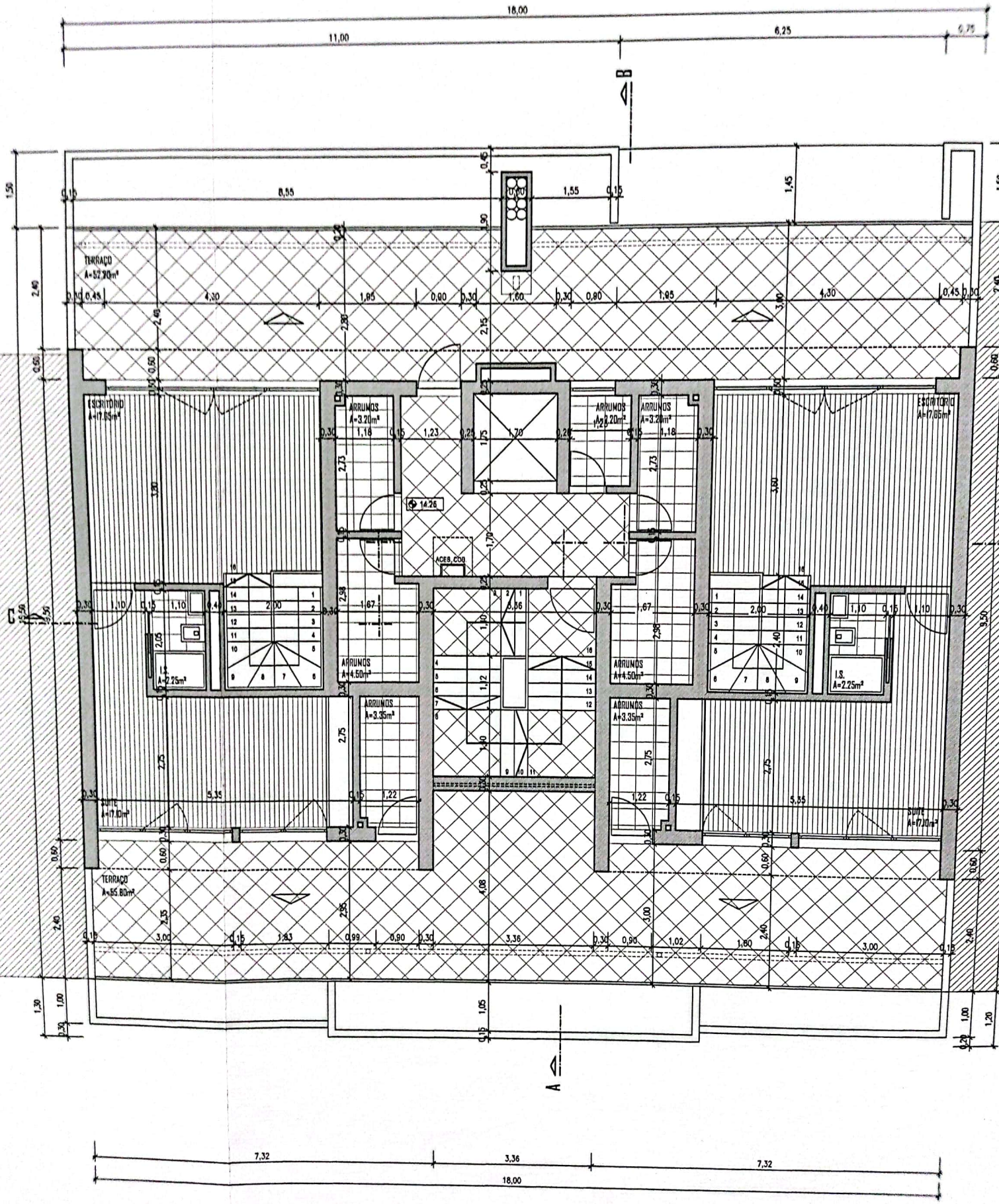
PLANTA SÔTÃO
